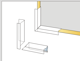
Snijden van U-profiel voor binnenhoek
